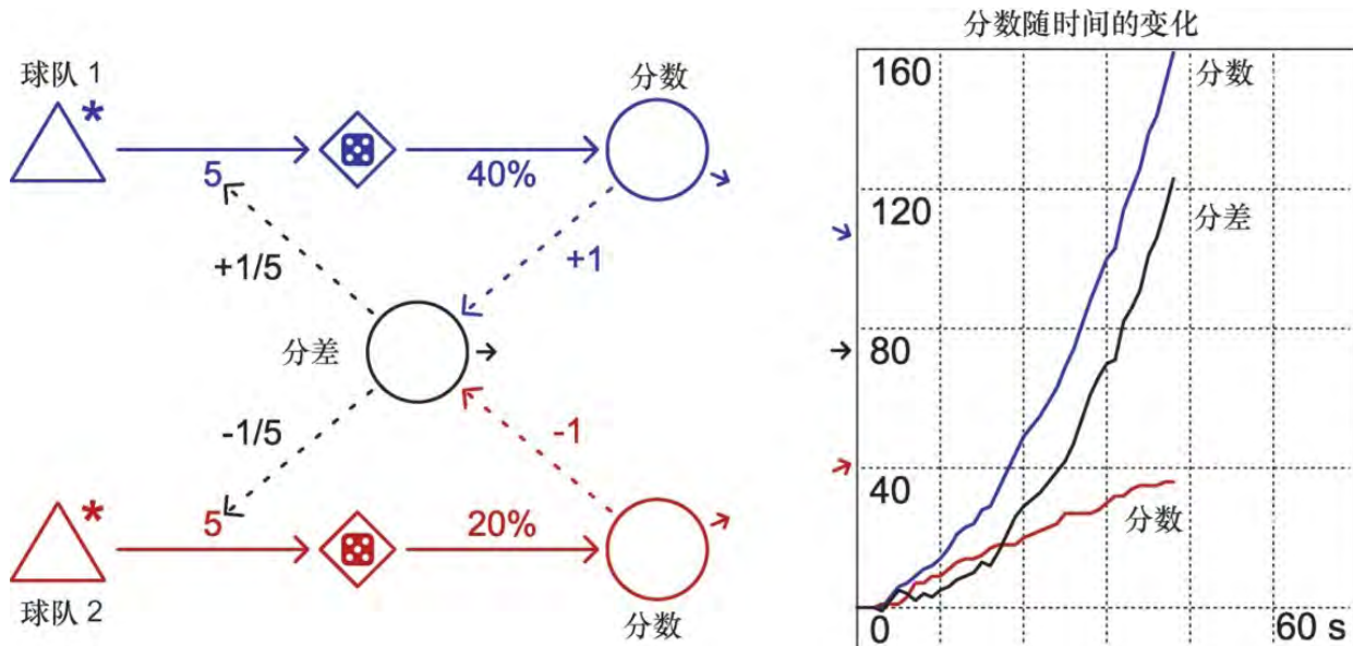
图6.21 正反馈篮球赛。我们需要在 Machinations 工具中将来源生产速率的最小值设置为 5，以防止出现某支队伍场上的少于5人的情况
