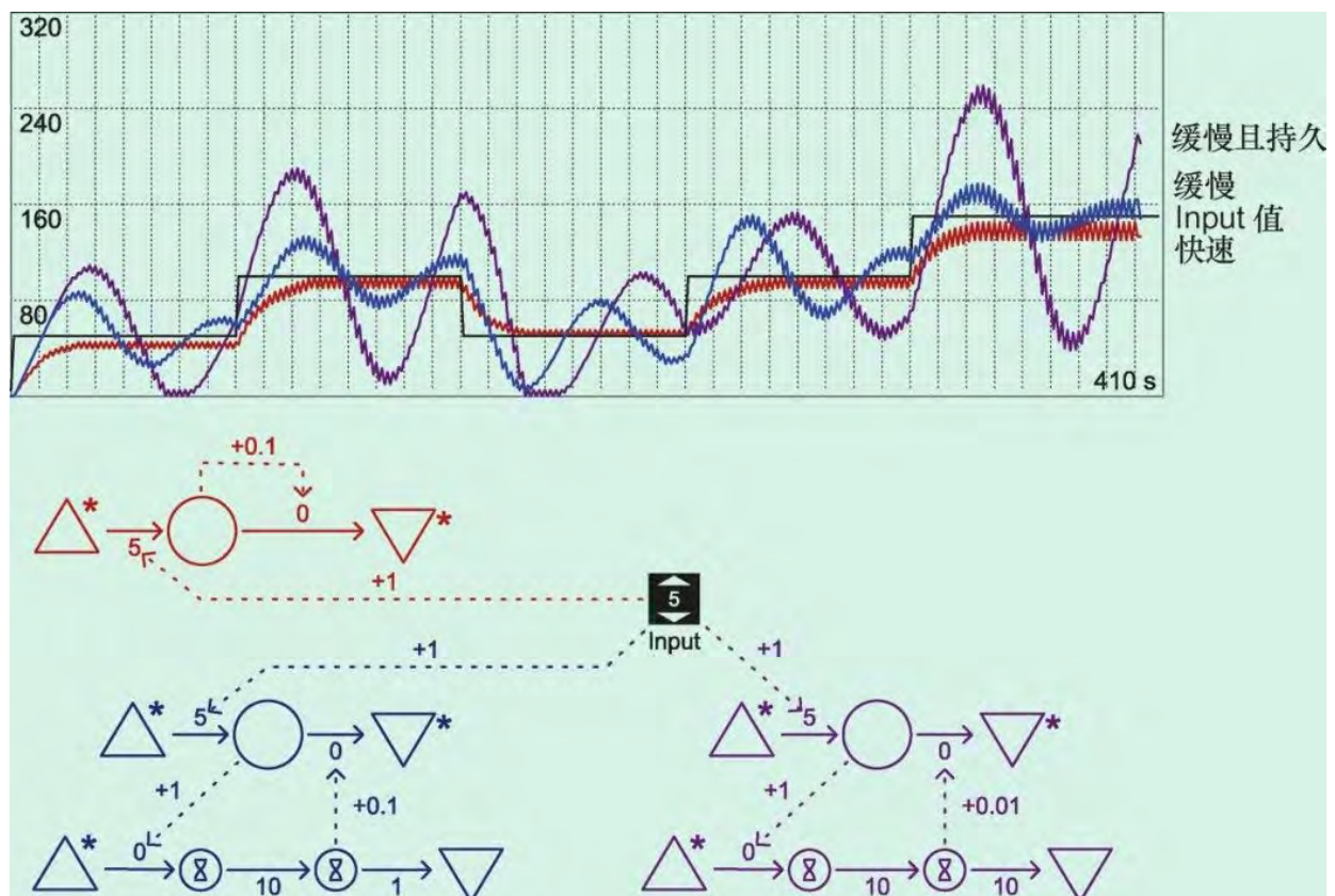
图9.6 负反馈变得更加缓慢和持久后的效果
