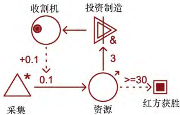
图6.31 一个简单的资源采集游戏。这个游戏是确定性的，红方总能获得胜利
