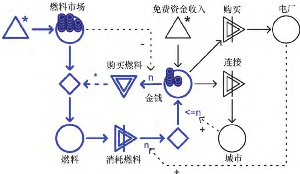
图B.5 《电力公司》中的生产机制。转换引擎用蓝色标示
