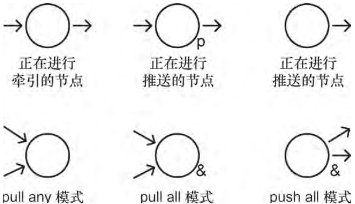
图5.7 各种牵引和推送模式
