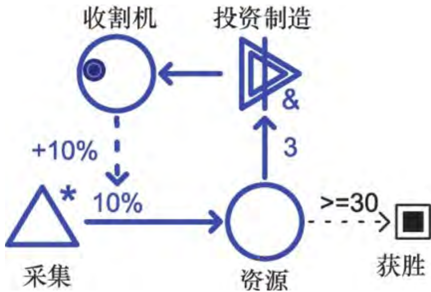
图7.2 资源采集游戏
