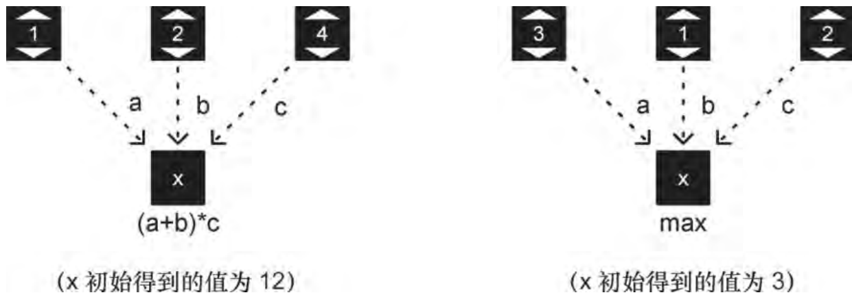
图6.2 用被动寄存器进行计算
