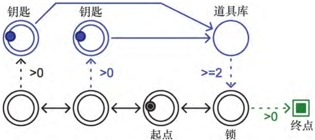
图11.8 一把需要多把钥匙才能打开的锁
