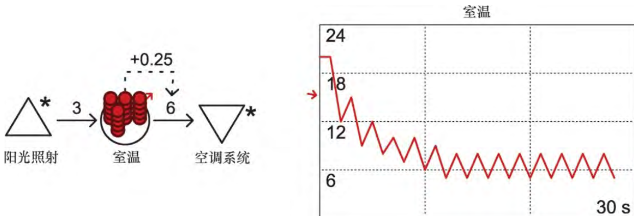
图6.19 用 Machinations 表现的空调系统
