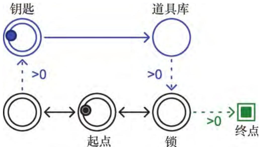
图11.7 一个简单的锁 - 钥匙机制（蓝色），用于控制玩家在游戏空间（黑色）中的进程
