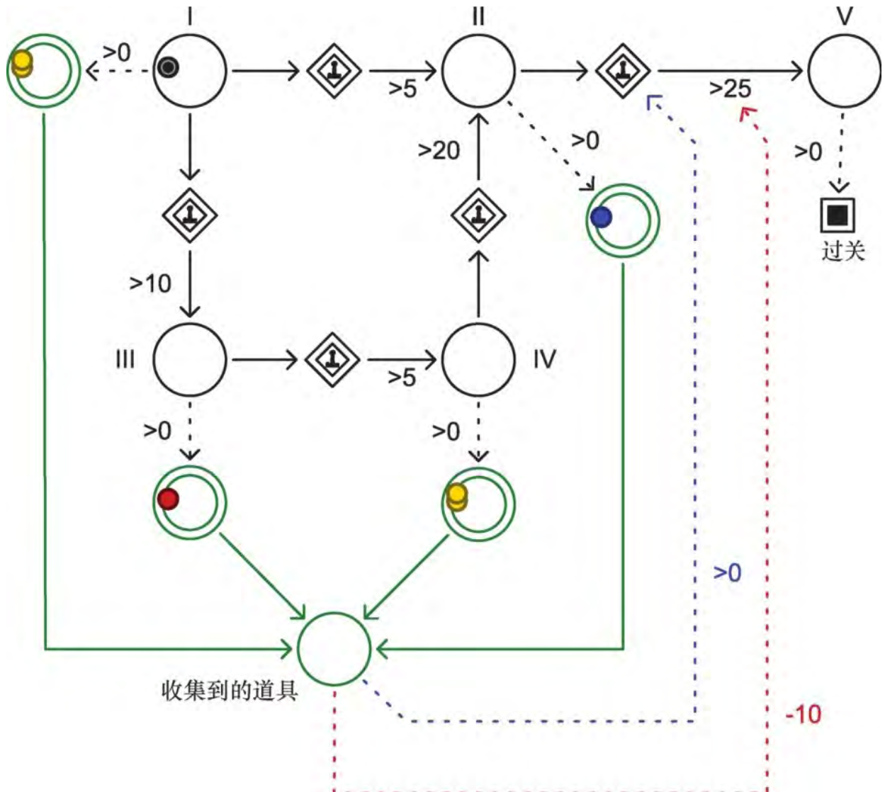
图6.34 玩家在一个动作游戏中四处收集增益道具的过程（此图省略了生命数的概念）
