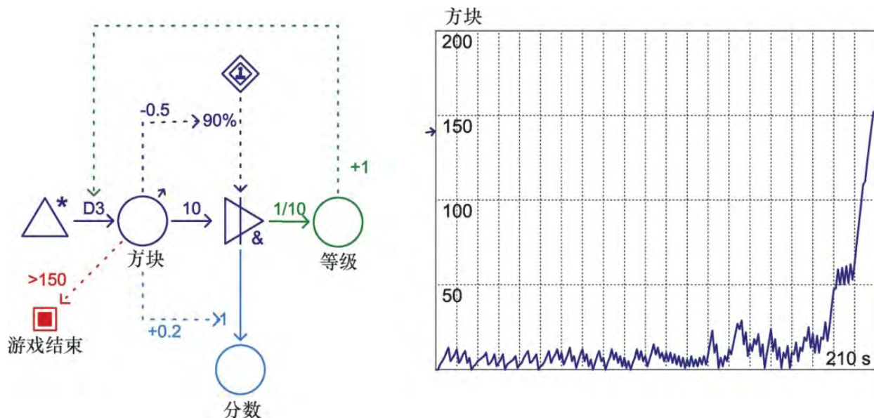
图B.13 《俄罗斯方块》中的渐增型复杂度
