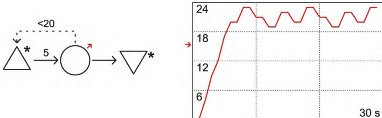
图6.17 应用了激活器的供暖反馈机制
