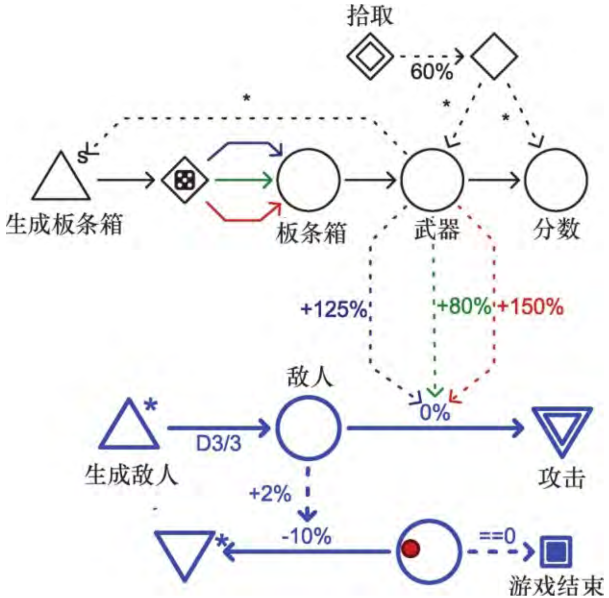
图B.14 《Super Crate Box》迫使玩家交替进行杀敌和捡箱子这两种行为
